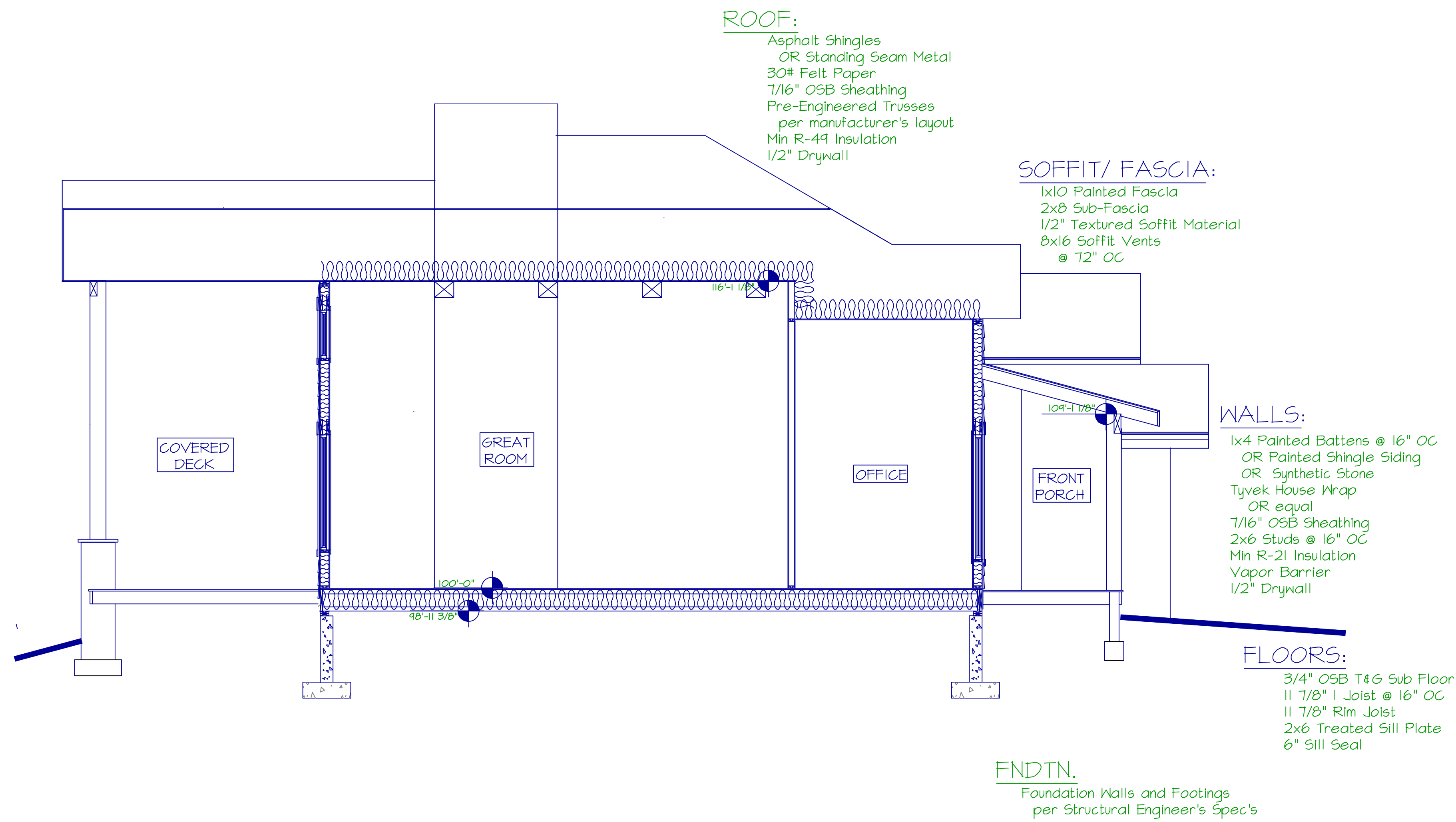
SECTION "A" SCALE: 3/16" = 1'-0"
